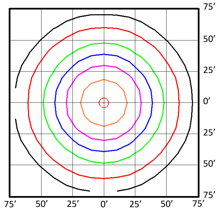
HBRE-21L-4K (20,859 Lumens)
