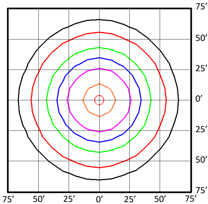
HBRE-14L-4K (14,497 Lumens)
