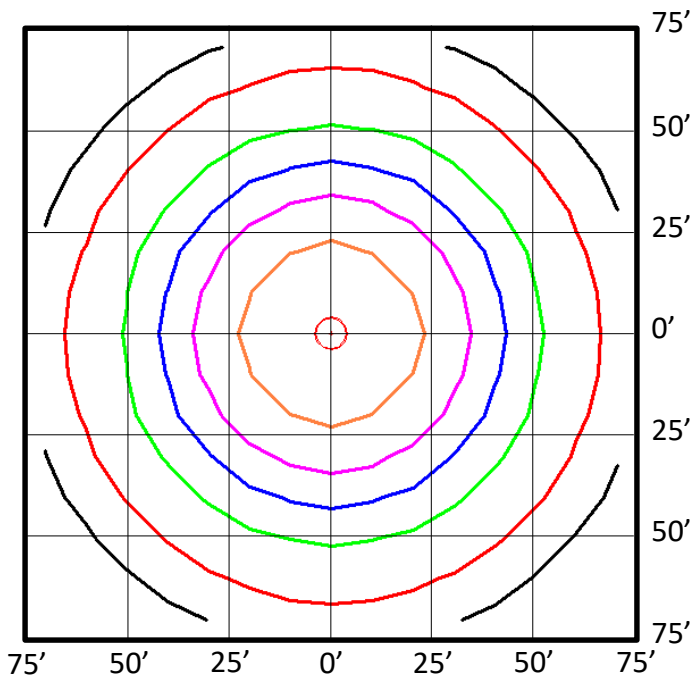
HBRE-28L-4K (28,341 Lumens)
